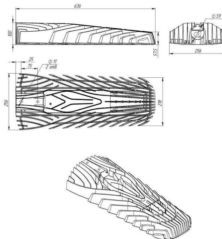
Рисунок 1 Габаритные размеры светильника «Superstreet 250», «Superstreet 340»
