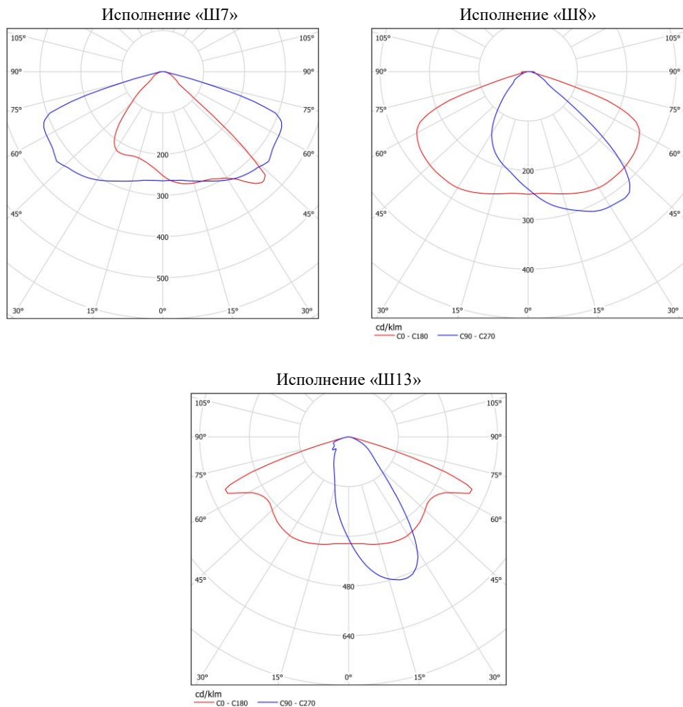
Рисунок 3 Типы КСС
